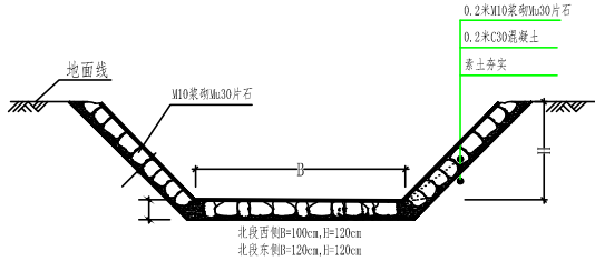
排水沟大样图
