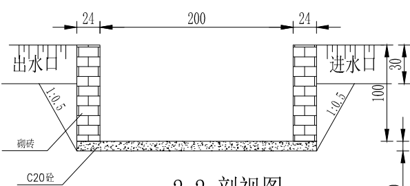
2-2 剖视图
