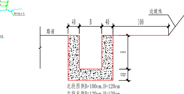
排水边沟大样
