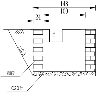
1-1 剖视图
