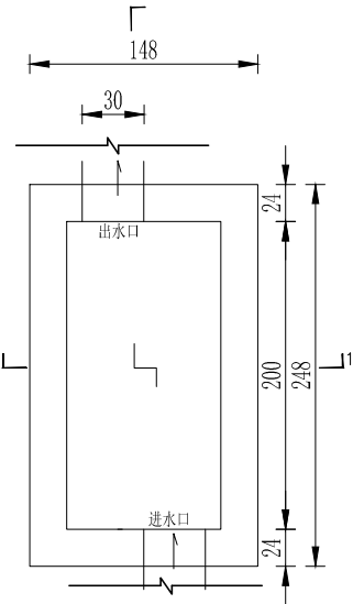
砖砌沉沙池平面图
